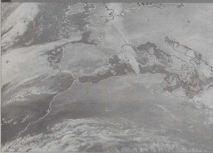
METEOSAT. IMAGEN TOMADA A LAS 17:00 HORAS DE AYER
