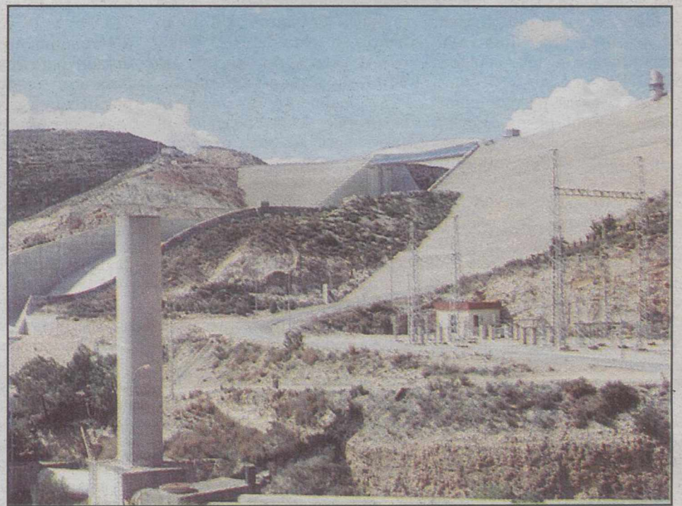
A la izquierda de la presa el aliviadero de Tous con una capacidad de desagüe de 19.700 m 3 /s.
