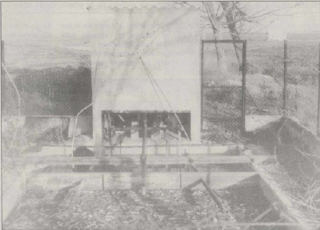
La depuradora de la Unidad Residencial Rehabilitadora de Las Tiesas.
