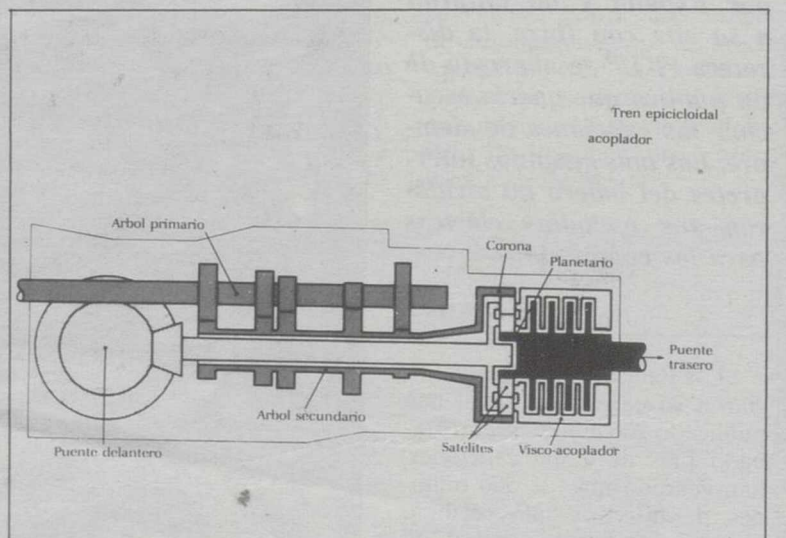
Esquema de la caja de cambios donde se aprecia el visco-acoplador.
