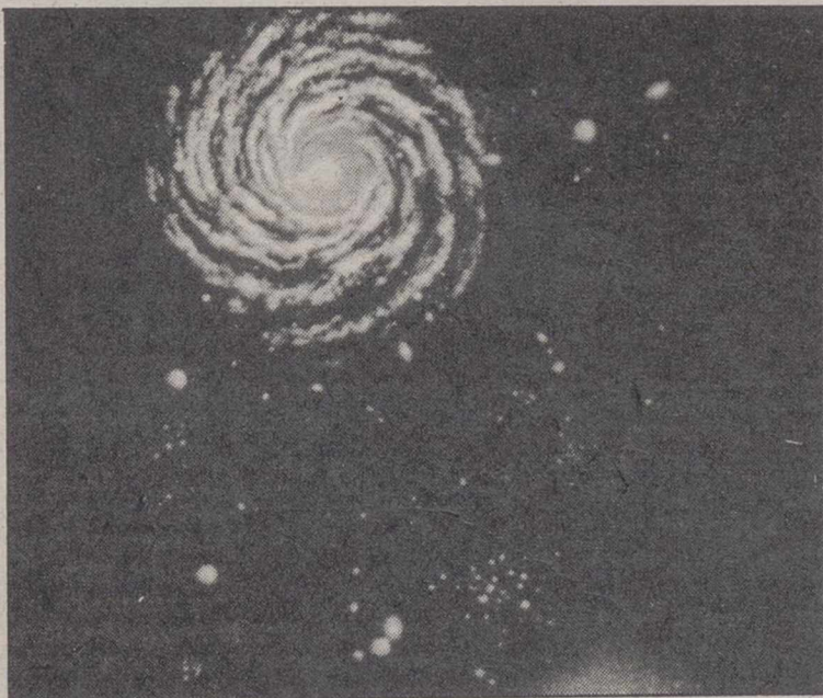
Se cree que el «Big Bang» originó el Universo.
