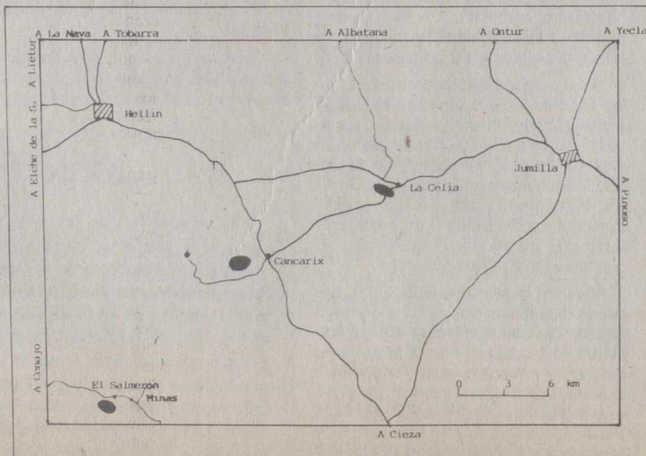
Mapa de la incidencia de las cordilleras Béticas en la región.
