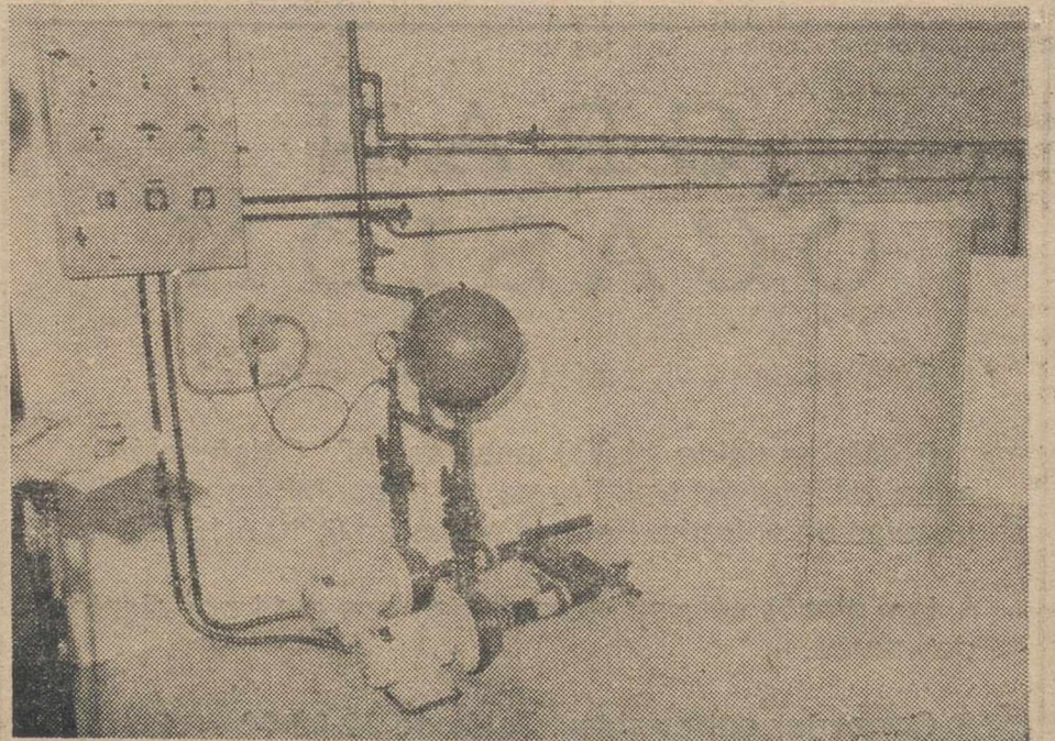
Depuradoras para la descalcificación y desionización de aguas.
