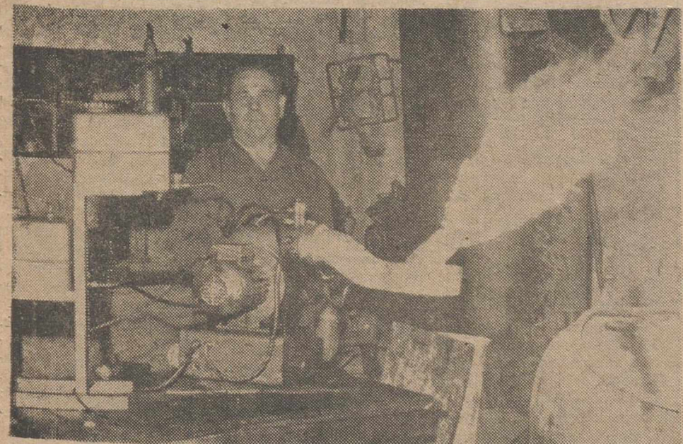
MALAGA.—Don Antonio Alvarez Rodriguez, malagueño, con su nuevo invento, ya patentado. Se trata de un quemador, con utilización en las industrias que en vez de usar gasolina, emplearía el aceite, ya quemado por los automóviles y que normalmente se tira, y consume de 7 a 9 litros por hora; mientras que los que hoy se utilizan gastan, nada menos que unos 30 litros de combustible.—(Foto EUROPA PRESS)
