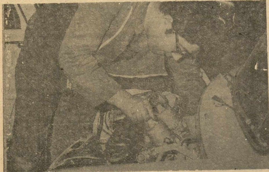
Una de las primeras fases de la transformación de un motor: el cambio de carburador. En la foto, un momento de la instalación de un doble carburador en "mini". (HISPANIA PRESS)
