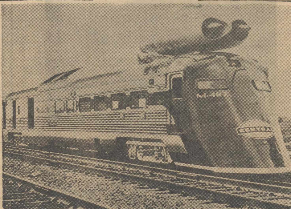
EISPKYNER (Ohio).—La locomotora completamente revolucionaria, a reacción, que ha hecho su viaje de pruebas entre Butler (Indiana) y Etstryner (Ohio), alcanzando los 275 kilómetros por hora. Ha sido probada por la compañía de ferrocarriles "New York Central". (Foto EUROPA PRESS)
