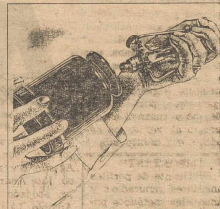
Enroscar el aparato a fondo con el fin de conseguir la perforación del cartucho y la salida del gas butano al cuerpo del grifo. En ningún caso, se desmontará el cartucho acoplado al aparato, hasta tanto no esté totalmente vacío.
