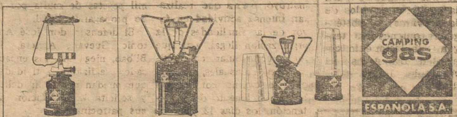
LUMIGAS "C" Altura: 30 cms. Diam.: 10 cms. MINIGAS "S" Altura: 20 cms. Diam.: 9 cms. MINIGAS "L" Altura: 24 cms. Diam.: 10 cms. Pesa: 310 grs. Consumo: 200 grs. por hora. Pesa: 415 grs. Consumo: 50 grs. por hora. Pesa: 580 grs. Consumo: 50 grs. por hora.
