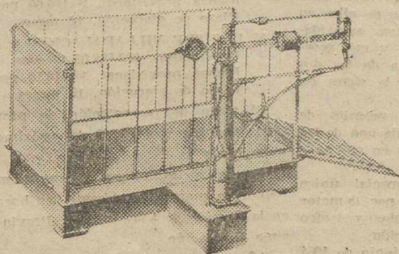
Báscula portátil para pesar ganado vivo
