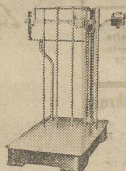
Báscula especial para pesar sacos
