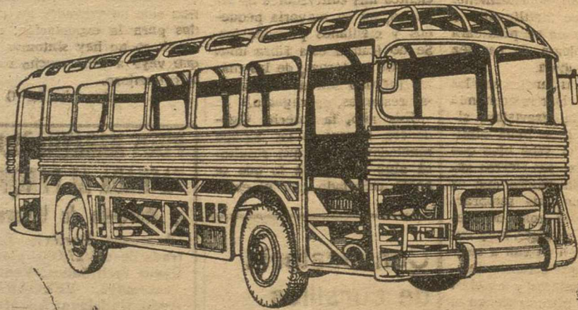
AUTOBASTIDOR: ESTRUCTURA MONOCASCO
