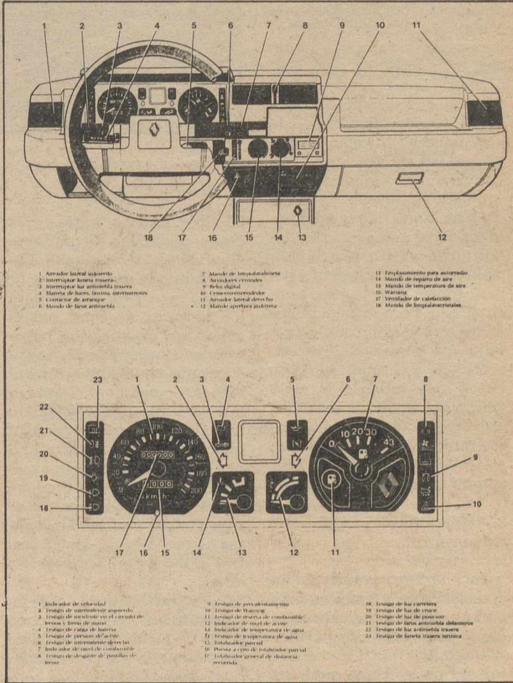
El salpicadero del Renault 5 Diesel—el mismo de los modelos de gasolina— es de una presencia muy agradable y un cuidado acabado. En detalle, la instrumentación de su cuadro.
