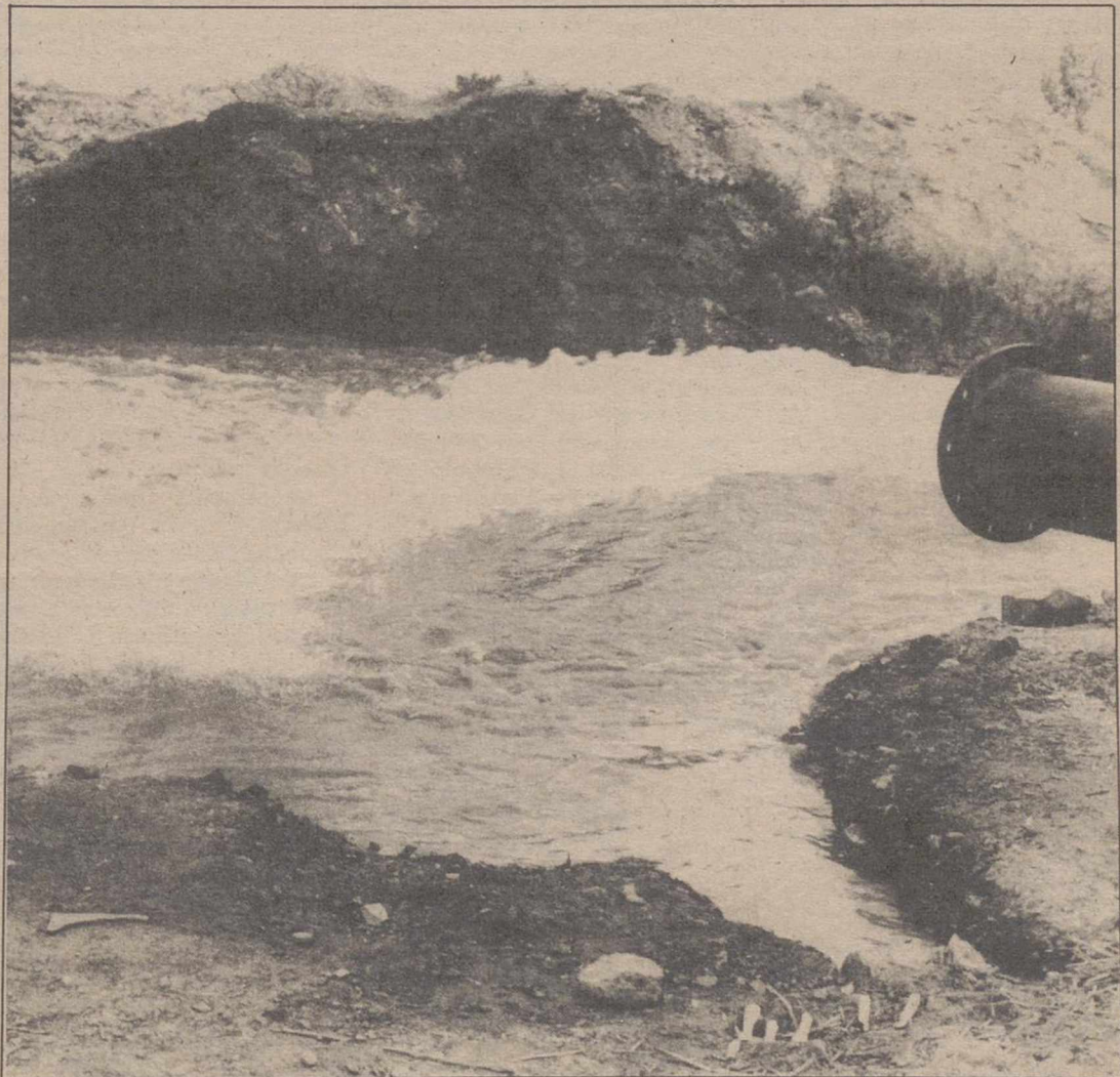
Vista de la sección del tubo, el cual posee una anchura de 250 milímetros de diámetro. En la fotografía se puede apreciar la presión del agua extraída y el caudal de 200 litros por segundo.
