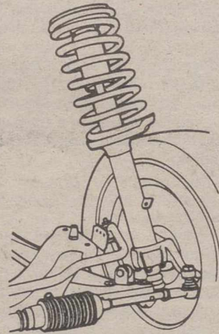
Principio del brazo elástico.
