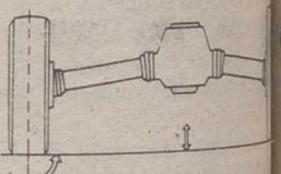
Suspensión trasera independiente con articulaciones en los ejes interior y exterior de los palieres. Ángulos de ruedas constantes, pero la altura libre sobre el suelo varía.
