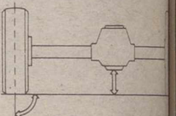
Eje trasero rígido. Ángulos de las ruedas, vía y altura libre sobre el suelo constantes.
