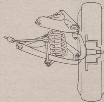
Suspensión delantera en dos brazos desiguales.
