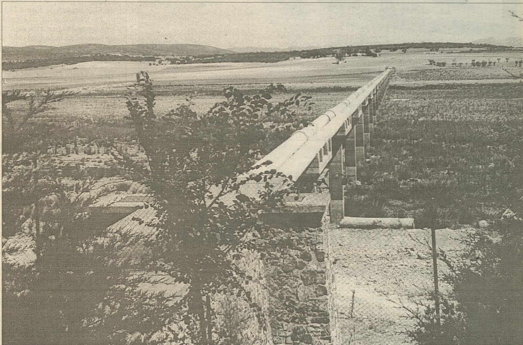
En la fotografía, el canal de agua procedente del embalse de Gasset que atraviesa bajo tierra el Club de Campo.
