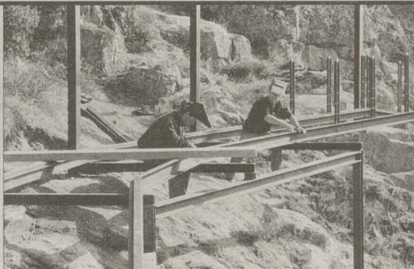
Pasarela peatonal. Los alumnos han construido una pasarela junto a la casa para no cerrar el camino que circula por la zona. / L.T.
