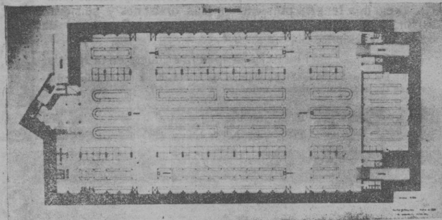
Plano general del proyecto de Mercado en la Plaza del Olivar, del arquitecto Sr. Forteza
