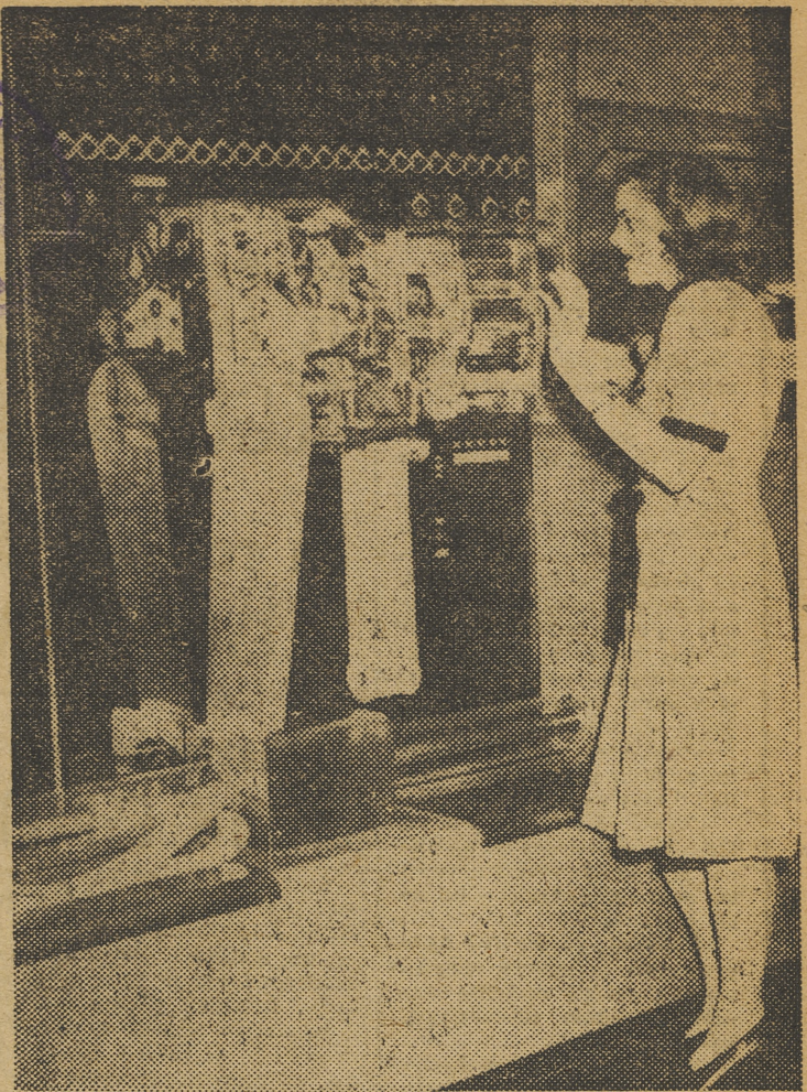
La mayor máquina calculadora del mundo, que empezó a construirse en 1945 en la Universidad de Harvard, está ahora realizando sus últimas pruebas y será entregada a la Marina norteamericana, en el mes de junio próximo. El cerebro mecánico, como se la llama, puede resolver, en un segundo, problemas de multiplicaciones sobre billones y es capaz de resolver problemas matemáticos casi demasiado complejos para la mente humana. Encierra un millón de pies de cable y ocupa una habitación de cincuenta por sesenta pies. — (Foto Ortiz)
