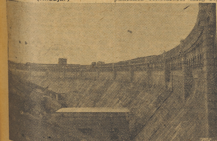
Una vista del pantano de La Cuerda del Pozo, inaugurado por los Ministros Secretario del Partido y de Obras Públicas, señores Arrese y Peña, en octubre de 1941
