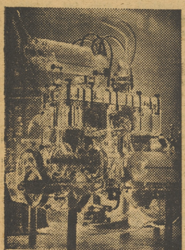
He aquí uno de los motores de cristal que ha sido inventado y construido en Alemania. (Foto Orbis)
