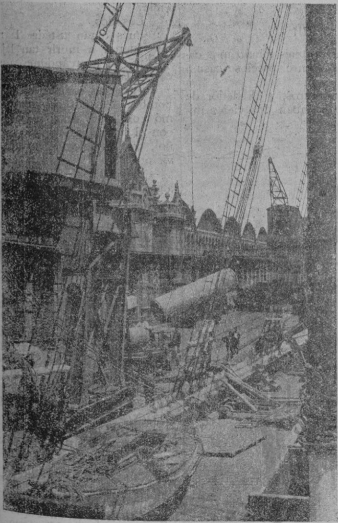
Embarque de los tubos para la canalización de las aguas
