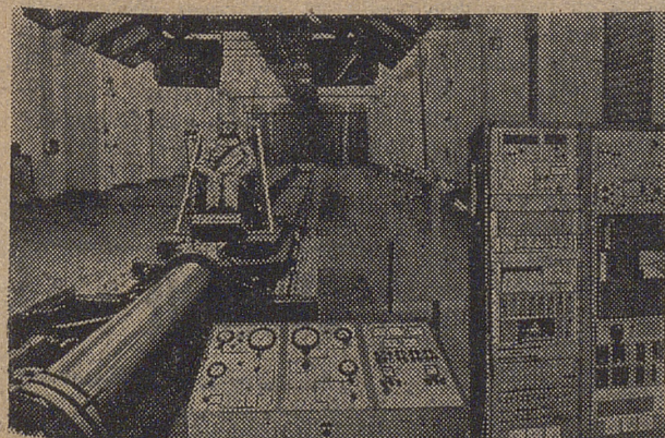
Túnel interior de pruebas, dotado de pistón neumático, zona reservada de seguridad y experimentación; se filma a 1.000 imágenes por segundo.
