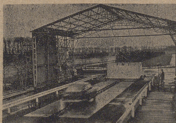
Pista exterior y túnel de pruebas accionado por pistón neumático.
