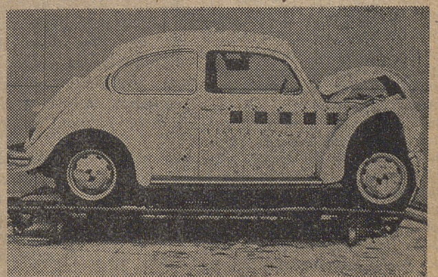
Golpe producido en el pistón neumático a una velocidad equivalente a 50 kilómetros por hora; prueba de parabrisas, y resistencia de materiales.
