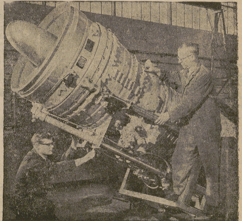
El primer turboalternador auxiliar de turbina de gases, de 15/18 megavatios. El alma del turboalternador es este motor de acuerdo con
