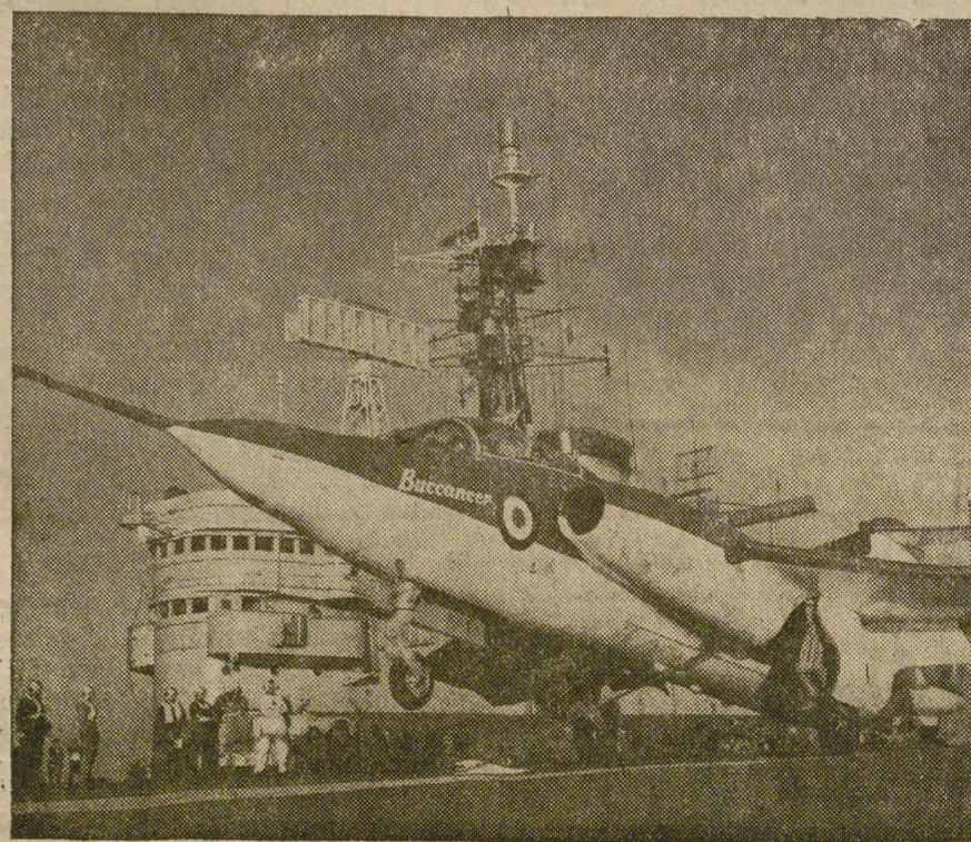
Este avión «Buccaner» está sobre la plataforma del portaaviones Ark Royal. Tiene dos plazas y aventaja a cualquier otro en el ataque a bajo nivel.
