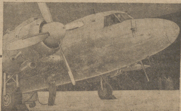
Magnífico bimotor «Viking» puesto a la disposición de los soberanos británicos en su viaje a Africa del Sur. Tiene una capacidad para 24 pasajeros y su radio de acción es de 3.000 kilómetros
