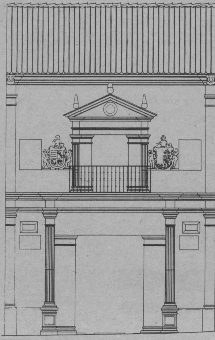
Alzado de la fachada principal del inmueble
