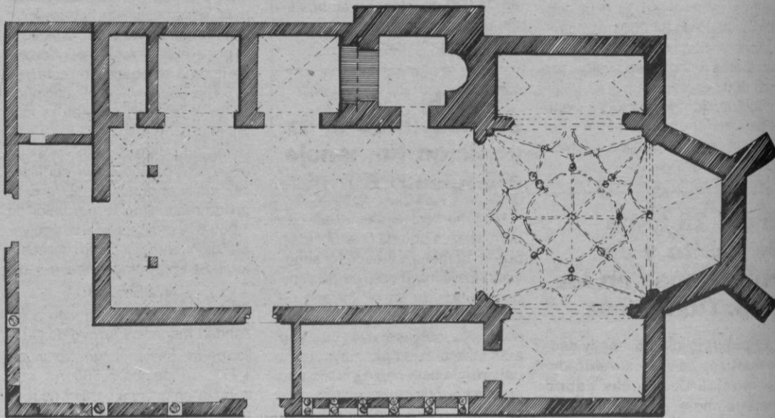
Planta de la iglesia de San Salvador
