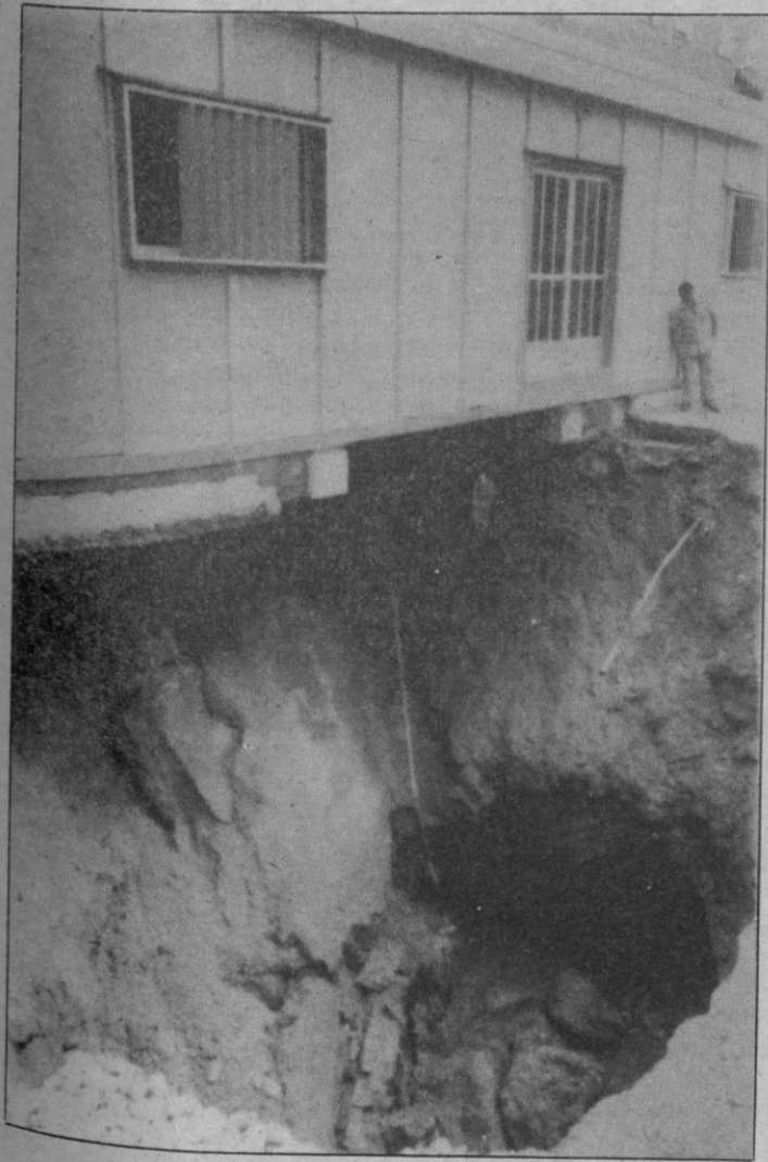
En el Polígono de San Millán en uno de sus patios donde están ubicadas unas aulas prefabricadas se produjo este socavón que dejó prácticamente en el aire a una de las aulas. El socavón lo provocó el río Clamores que pasa por debajo
