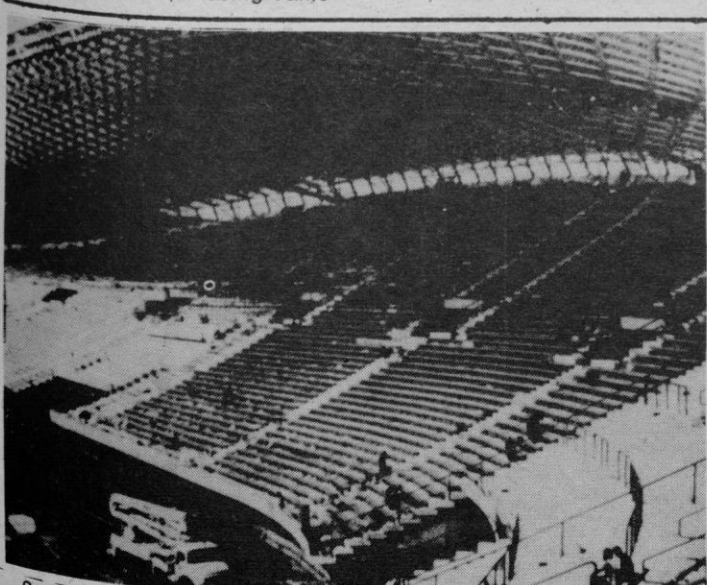
Semejante a una gigantesca concha se extiende el techo de la tribuna del nuevo estadio de Split (Yugoslavia). Las principales características son: 200 metros de extensión sin columnas, 45 metros de volada y 39 de altura sobre el terreno de juego. Unos 6.500 tirantes de acero, sujetos por casi 1.700 soportes, mantienen el techo, diseñado y desarrollado por la empresa Mero, en la que participa el consorcio Mannesmann, de la República Federal de Alemania. (Foto: did/Mannesmann)
