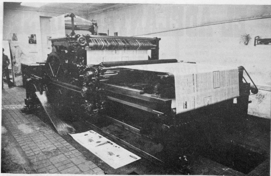
He aquí a la auténtica «heroína» del antiguo sistema de tipografía. Hace cincuenta años que entró en servicio esta rotoplana, en la que EL ADELANTADO DE SEGOVIA ha venido tirándose. Ningún día quedó sin salir el periódico por fallo de esta máquina.
