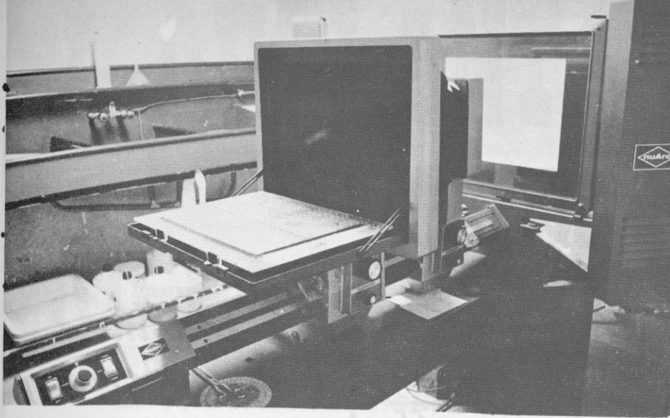
Mientras se preparan las maquetas, en el laboratorio fotográfico se revelan las fotos, que pasan luego a las maquetas y éstas son fotografiadas a su vez, completas, en la cámara del presente grabado.
