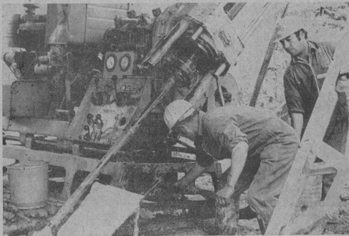
Tapia de Casariego.—Esta es una de las máquinas que realizan sondeos auríferos en la provincia de Oviedo, donde ya se han descubierto importantes yacimientos de este metal; concretamente en el término de Tapia de Casariego.—(Foto Europa Press)
