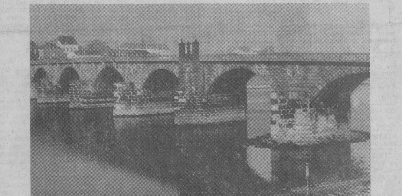
Tréveris.—Alrededor del año 200 después de J. C., los romanos construyeron este puente de 350 metros de longitud cerca de Tréveris, en el Oeste de la República Federal de Alemania, sobre el río Mosela. Aunque con ocasionales trabajos de reparación, este puente sigue sirviendo en su estado primitivo para el moderno tráfico en masa. Los sillares sobre los siete pasos parecen ser ensamblados para la eternidad. Técnica y arquitectónicamente, el puente representa una obra maestra. Los fundamentos de los pilares descansan en el cauce hasta a una profundidad de más de veinte metros.—(Foto DaD.)
