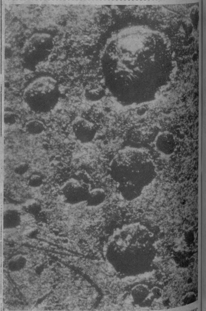
Mulhouse (Francia).—Esta fotografía muestra el perfecto resultado conseguido en la simulación del impacto de los meteoritos en el suelo lunar. Ha sido conseguido mediante disparo de pequeños proyectiles a gran velocidad sobre una placa de aluminio.—(Foto Europa Press)
