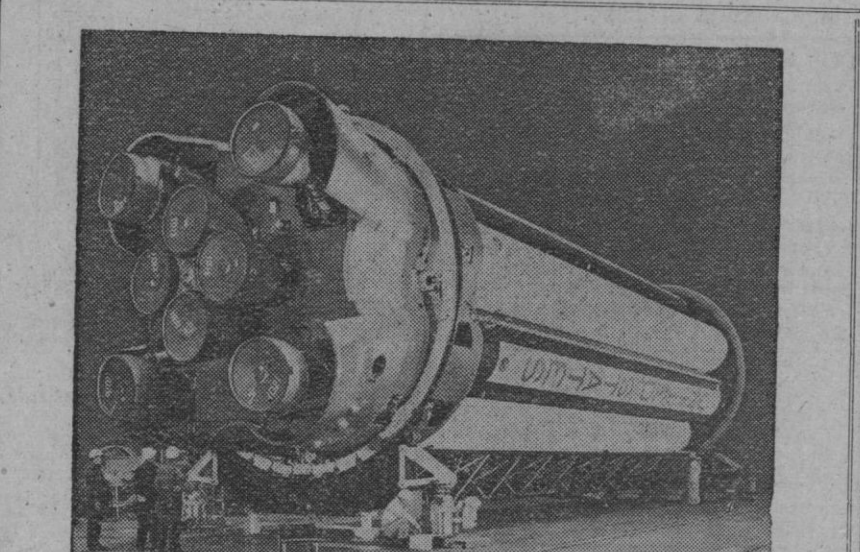
La primera fase del vehículo portador Saturno es de proporciones tan gigantescas que a su lado los hombres parecen enanos. Este cohete acelerador se está construyendo en el Centro de Vuelos Espaciales Marshall, de Huntsville, Alabama. Se utilizará para colocar en órbita la primera astronave con tripulación múltiple y para llevar al espacio modelos avanzados, situarlos en órbita alrededor de la Luna y hacerlos desembarcar en ella
