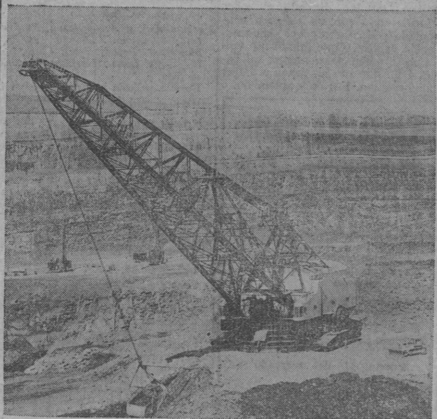
Moderna pala de arrastre que ha comenzado a usarse en mineras de cielo abierto en Gales. Construida con un costa de novecientos mil libras esterlinas se dice es la mayor de Europa y una de las más grandes del mundo. Aparece funcionando en la parte superior del gráfico. La topadora a la mano derecha da idea de su gigantesco tamaño. La fotografía inferior muestra uno de los dos inmensos cangilones. Ese solo pesa 34 toneladas y mide 5,85 metros de largo, 4,12 metros de ancho y 4,35 metros de altura. La pala de arrastre funciona con dos secciones de botolón. El botolón de 86,4 metros tiene una carga de trabajo de 65 toneladas, a su radio máximo de 78 metros, pudiendo descargar desde 39 metros de distancia. El botolón más pequeño, de 74,1 metros, puede levantar 91 toneladas de peso a su radio máximo de 69 metros, pudiendo descargar desde 30. Los cangilones recogen 23 y 30 metros cúbicos, respectivamente
