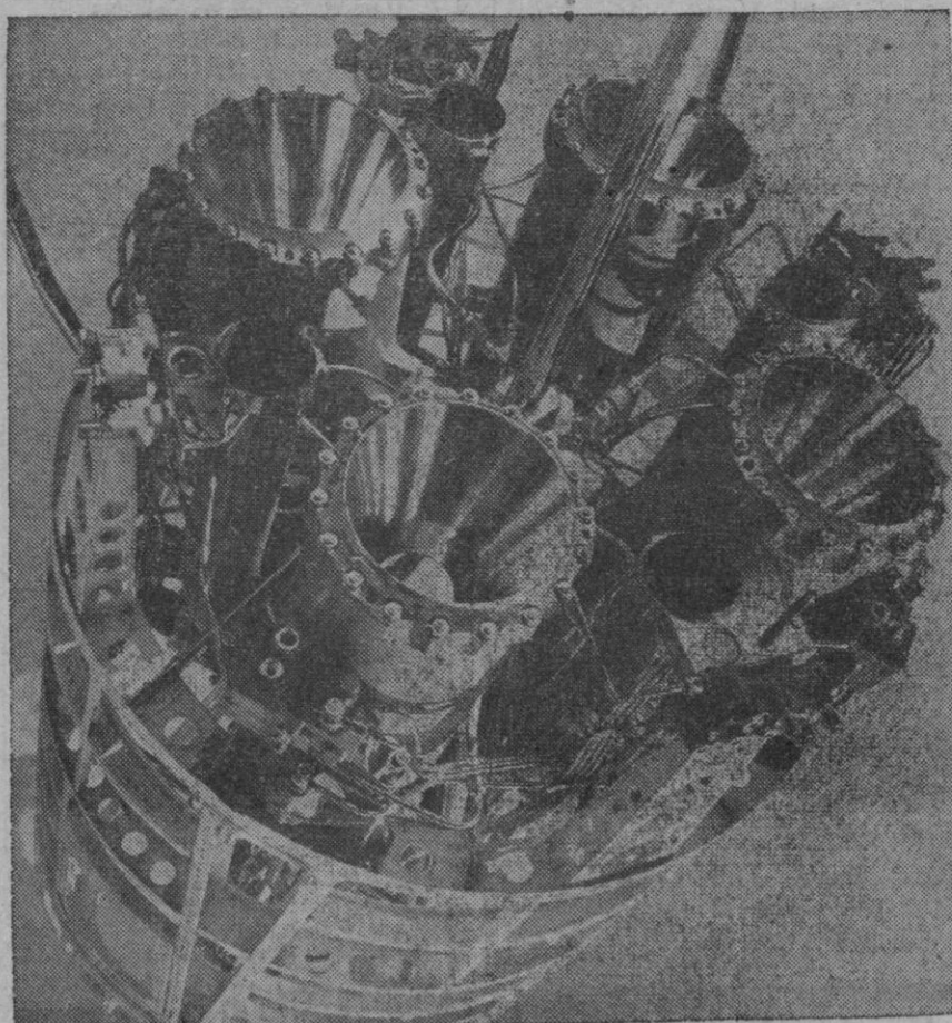
El Bristol Siddeley Gamma Mk 201, motor que propulsa los cohetes británicos Black Knight, proyectiles de investigación que retornan a la Tierra. En los cinco disparos sucesivos del Black Knight, hechos en el campo de tiro de Woomera, Australia, estos ingenios han llegado a alturas de entre los cuatrocientos y los ochocientos kilómetros, regresando a la Tierra en la zona prevista. Durante su vuelo, los Black Knight han registrado una velocidad diez veces superior a la del sonido. El motor del cohete citado, el cual, con su envoltura, pesa aproximadamente 317 kilogramos, tiene una reacción impulsora, a nivel de mar, de 7.440 kilogramos, que se eleva a casi diecinueve mil kilogramos fuera de la atmósfera terrestre. Los combustibles, que son peróxido de hidrógeno y keroseno, se queman en sus cuatro cámaras de combustión para dar dicho impulso de avance.
