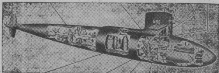
Este es un dibujo seccionado del USS Skipjack, que según sus constructores es "el submarino más rápido y maniobrero del mundo". Este barco, en forma de tiburón, cuyos rasgos revolucionarios incluyen una única hélice y planos de inmersión situados en la torre de mando, fue botado hace poco en Groton, Connecticut.
