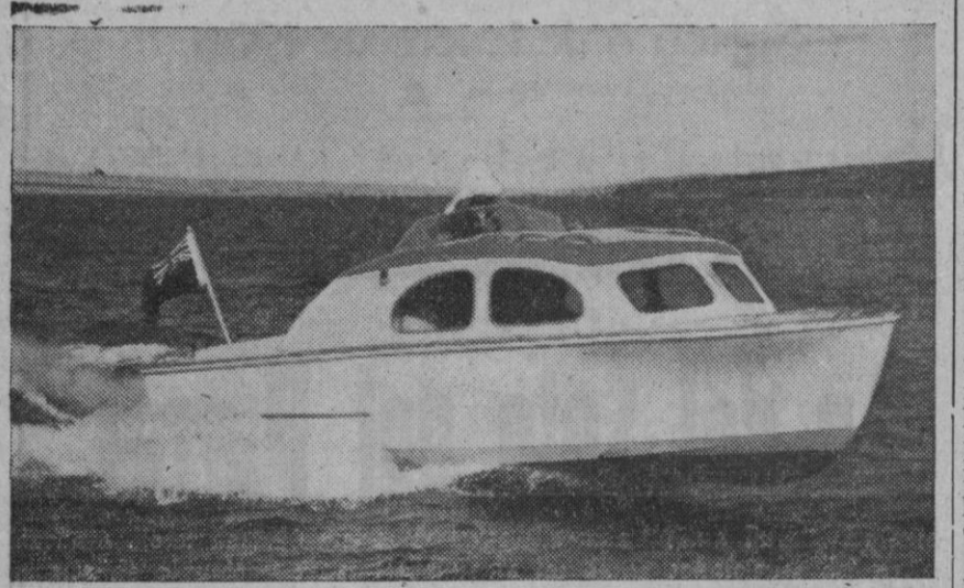
Lancha a motor de 7,20 metros de largo, llamada "Tuna Twin". Es enteramente de plástico y resiste igualmente las duras condiciones del Ártico que de los Trópicos. La embarcación, construida en Gran Bretaña, está moldeada de una sola pieza de resina poliéster reforzada con fibra de cristal. Carece de juntas, por lo que la filtración es imposible
