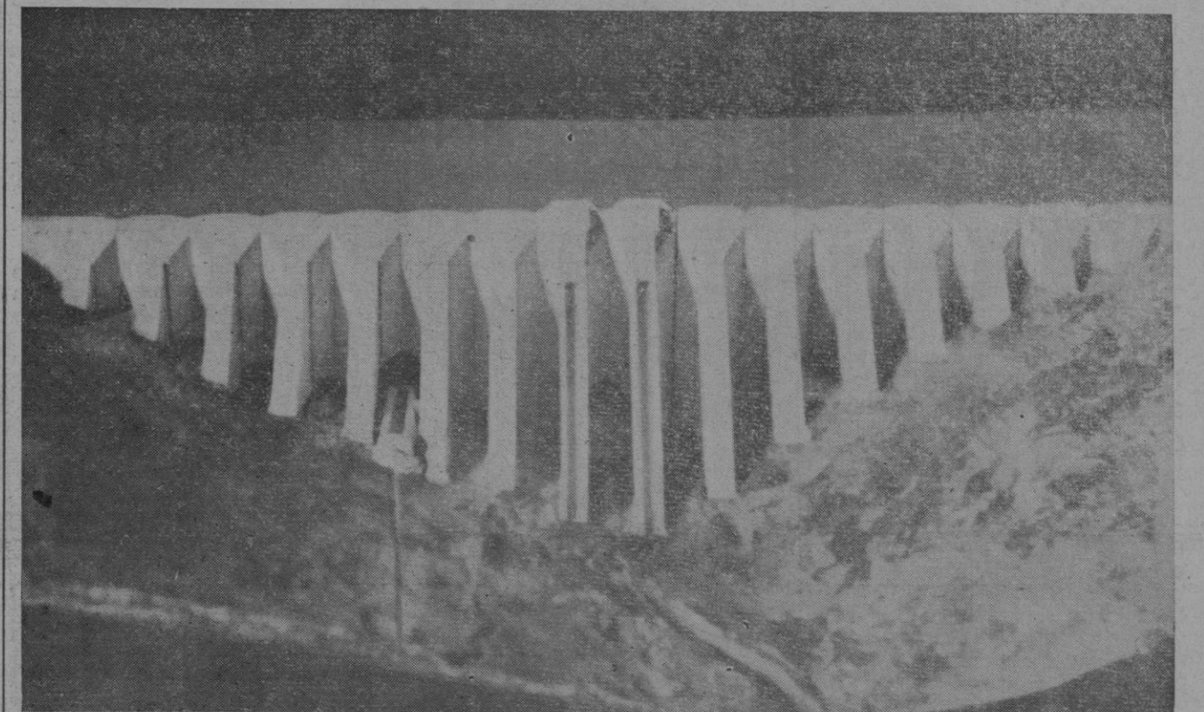
Un aspecto de la maqueta de la presa que, por el sistema de contrafuerte, se construirá en el término de Revenga, cerca de la curva de Puente Alta, de la carretera de San Rafael. Tendrá 38 metros de altura y 200 de longitud, siendo de 2.500.000 metros cúbicos la capacidad del embalse
