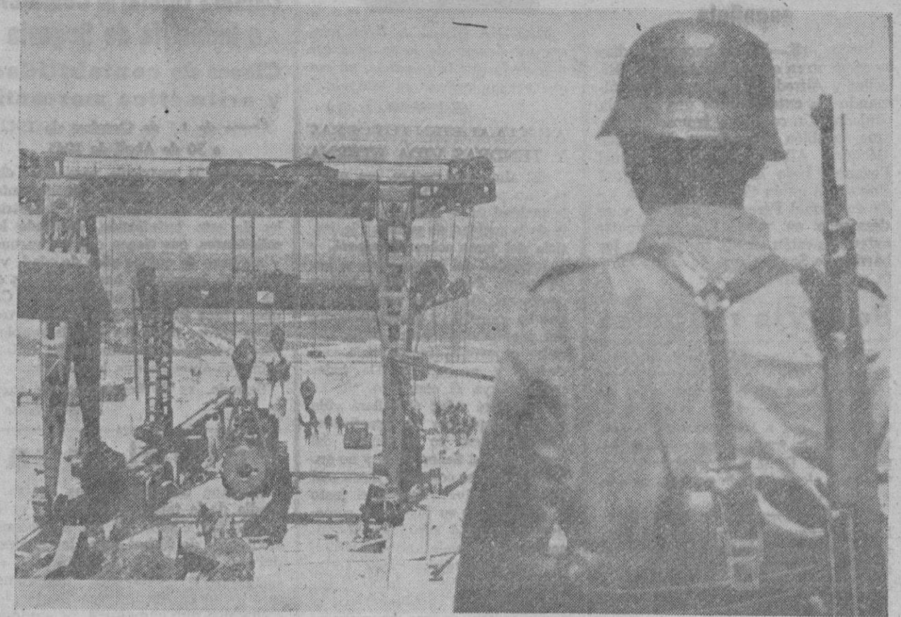
EN LA COSTA FRANCESA DE LA MANCHA.—Operación de montaje, por medio de grúas, de un tubo de cañón gigante alemán.
