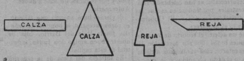
RECORTES Y PLETINAS PARA FABRICACIÓN DE HERRADURAS
