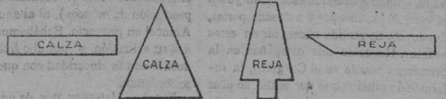
RECORTES Y PLETINAS PARA FABRICACIÓN DE HERRADURAS.
