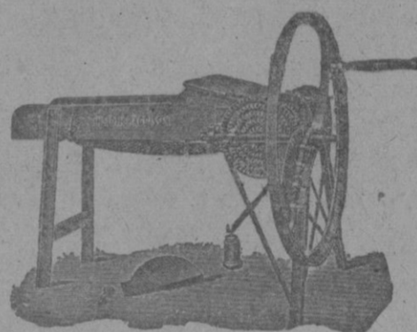
Corta Forrajes para Paja, alfalfa etc. automáticos y regulables para distintos cortes
