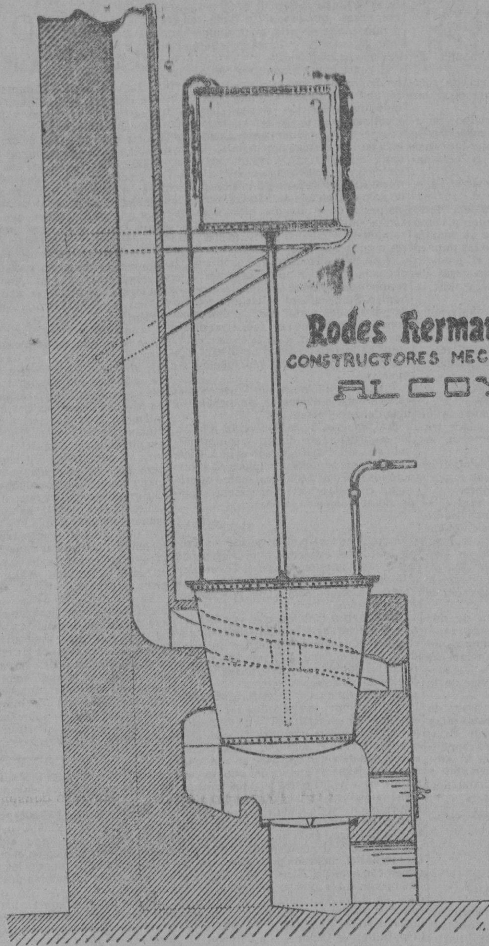
Aparato Termo-Sifón para aceite
