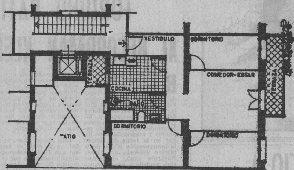
VIVIENDA TIPO VIRGEN DEL VAL (BARRIO DE LA CONCEPCION)
