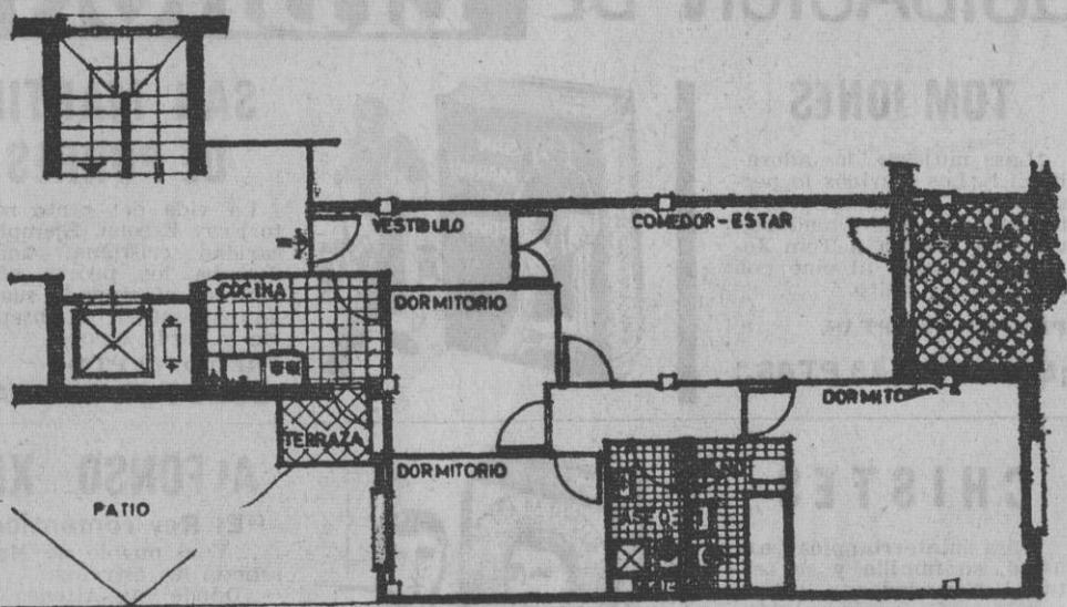
VIVIENDA TIPO RIOMANZANARES
