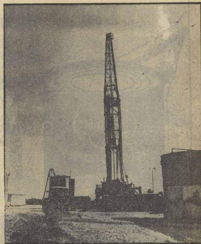
«Ayoluengo 12», a cargo de técnicos franceses. La torre es muy moderna, pero aún lo será más la que se instale en el «Ayoluengo 13». Las previsiones para este pozo parecen ser buenas.
