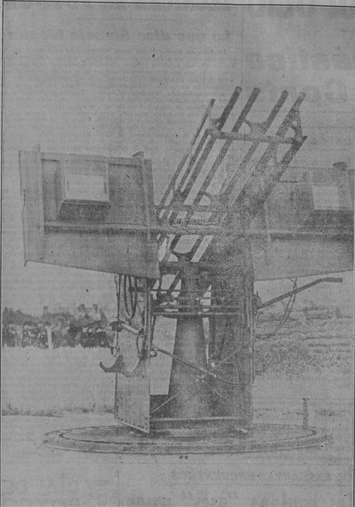
Por primera vez se publica la fotografía del lanzacohetes antiaéreo, arma eficazísima, probada ya con éxito en la actual guerra aérea. (Foto Gil del Espinar.)
