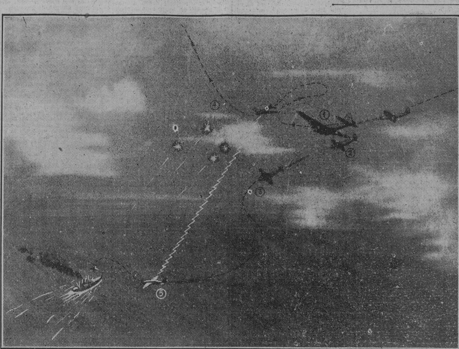
1. El "avión madre" remolcando uno o varios planeadores dirigidos. 2. El "avión madre" suelta la bomba planeadora cohete eléctrica. 3. El propulsor del cohete impulsa la bomba hacia el objetivo. 4. El "avión madre" vuela fuera del alcance de la D. C. A. y dirige por T. S. H. la bomba planeadora hacia el objetivo.
